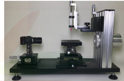
水滴角测试设备 Test machine for contact angles
