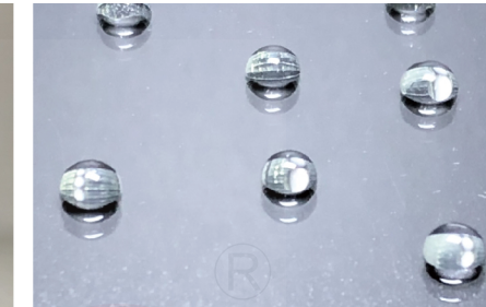
水滴角
